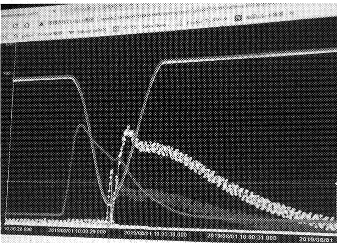
モニター画面では故障発生前後の加速度値(一番上の線)が変化
